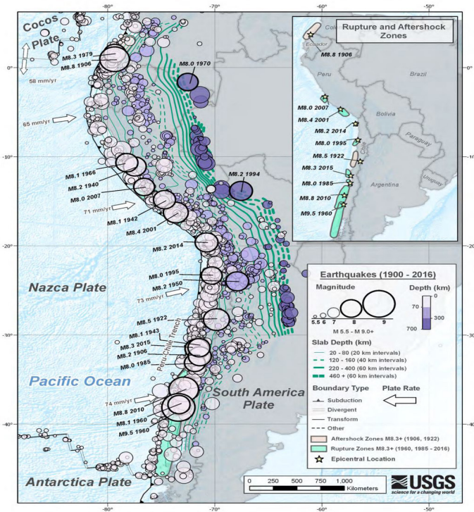
Figura 4. Sismos mayores a magnitud 5.5 ocurridos entre 1900 y 2016 a lo largo de la costa de Sudamérica tomada el 15 de agosto de 2023. Para los detalles ver el texto. Fuente USGS, 2023.
